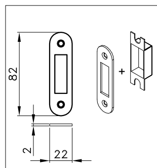
Prihvatnik-šild HCS-SB-E F 69 s podmetačem
