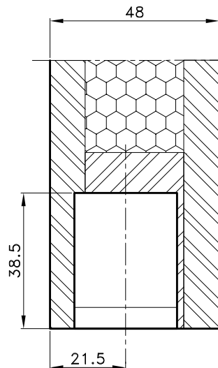
PRESJEK 2-2
