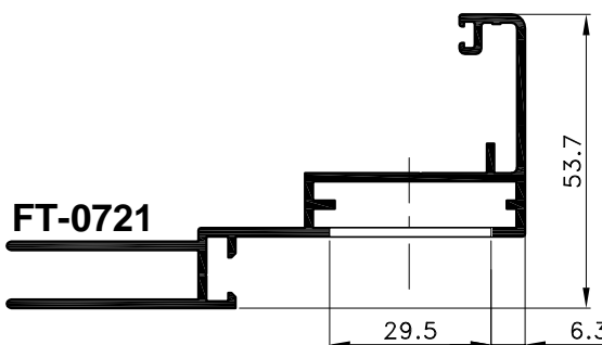
PRESJEK 1-1
