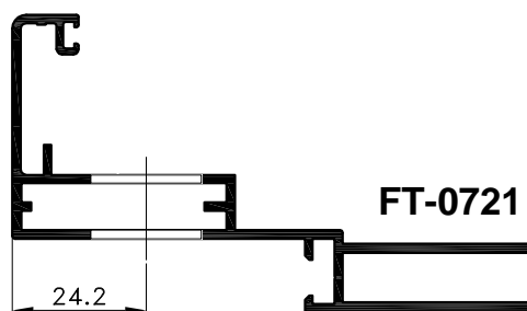
PRESJEK 1-1
