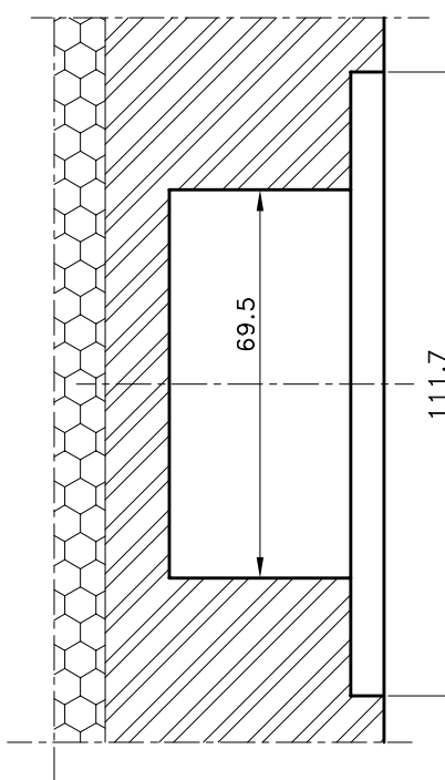
PRESJEK 3-3
