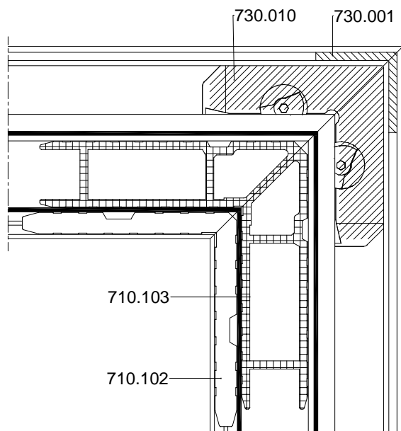
PRESJEK B-B
