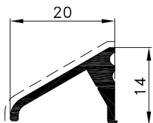
Z40-657 težina: kg/ml 0.186 svj.povr. mm 23
