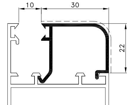
D45-041 težina: kg/ml 0.307 svj.povr. mm 50
