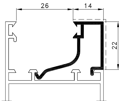
D45-042 težina: kg/ml 0.295 svj.povr. mm 36
