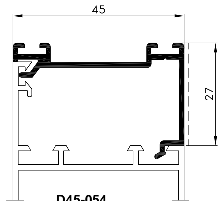
D45-054 težina: kg/ml 0.386 svj.povr. mm 32
