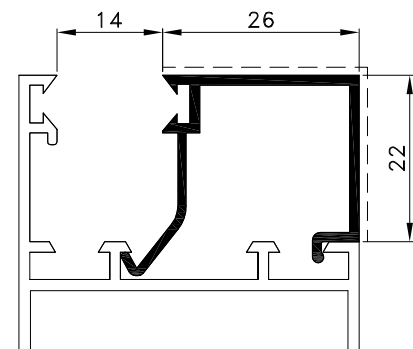
D45-045 težina: kg/ml 0.293 svj.povr. mm 48
