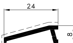
F-0228 težina: kg/ml 0.153 svj.povr. mm 27
