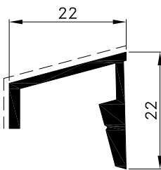
060 350 težina: kg/ml 0.285 svj.povr. mm 31
