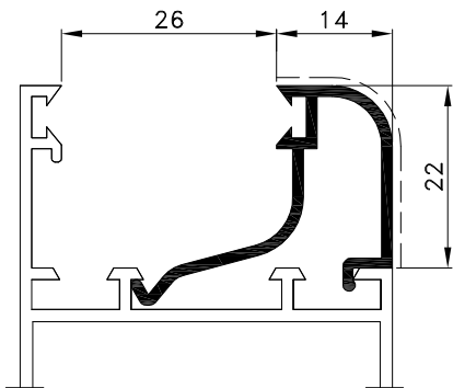
D45-040 težina: kg/ml 0.285 svj.povr. mm 34
