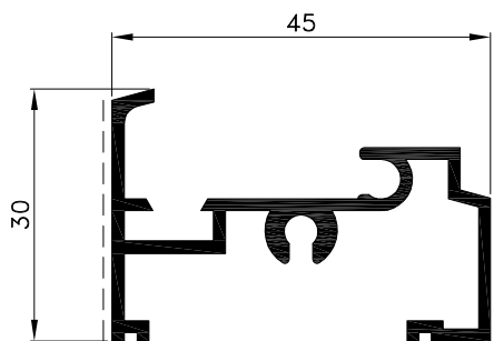
D45-050 težina: kg/ml 0.588 svj.povr. mm 46
