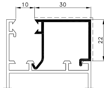
D45-043 težina: kg/ml 0.304 svj.povr. mm 52
