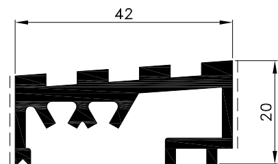
060 353 težina: kg/ml 0.825 svj.povr. mm 34
