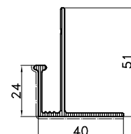
F-1132 tež.:0.567 kg/m'
