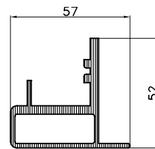
KF-020/22 tež.:1.377 kg/m'
