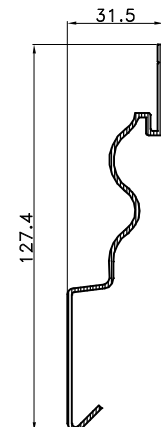
F-1126 tež.:0.704 kg/m'
