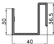
F-1130 tež.:1.60 kg/m'
