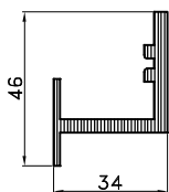
KF-020/21 tež.:0.895 kg/m'
