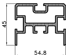
F-0798 tež.:1.55 kg/m'
