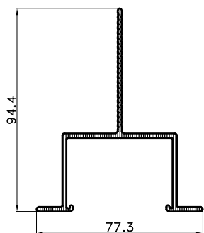
F-1120 tež.:1.160 kg/m'
