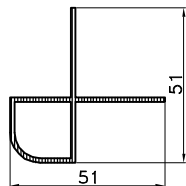
F-1125 tež.:0.545 kg/m'
