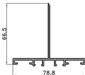
KF-001 tež.:0.964 kg/m'
