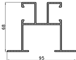
F-5-5-1 tež.:1.641 kg/m'
