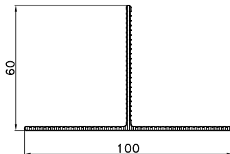
F-0934 tež.:0.78 kg/m'
