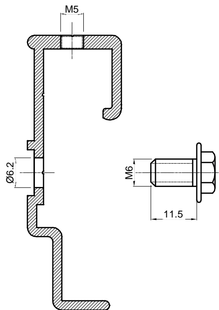
nosač trespe KS-T50
