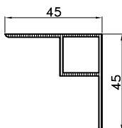
F-1124 tež.:0.477 kg/m'
