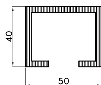
KF-022 tež.:1.55 kg/m'
