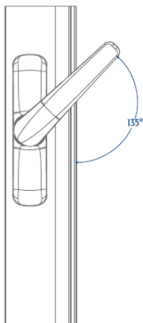
Pokretanje ručke
